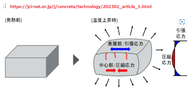
図-2 内部拘束による温度ひび割れイメージ図
